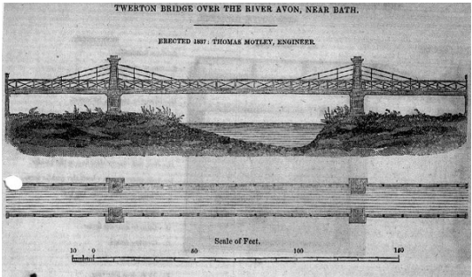
1837 Pont de Twerton (GB)
