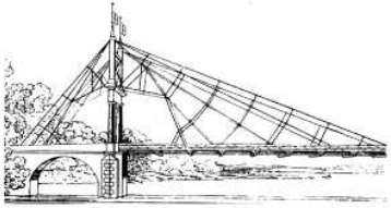
1824 Pont de Nienburg (D)
